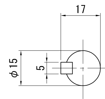
軸端寸法
